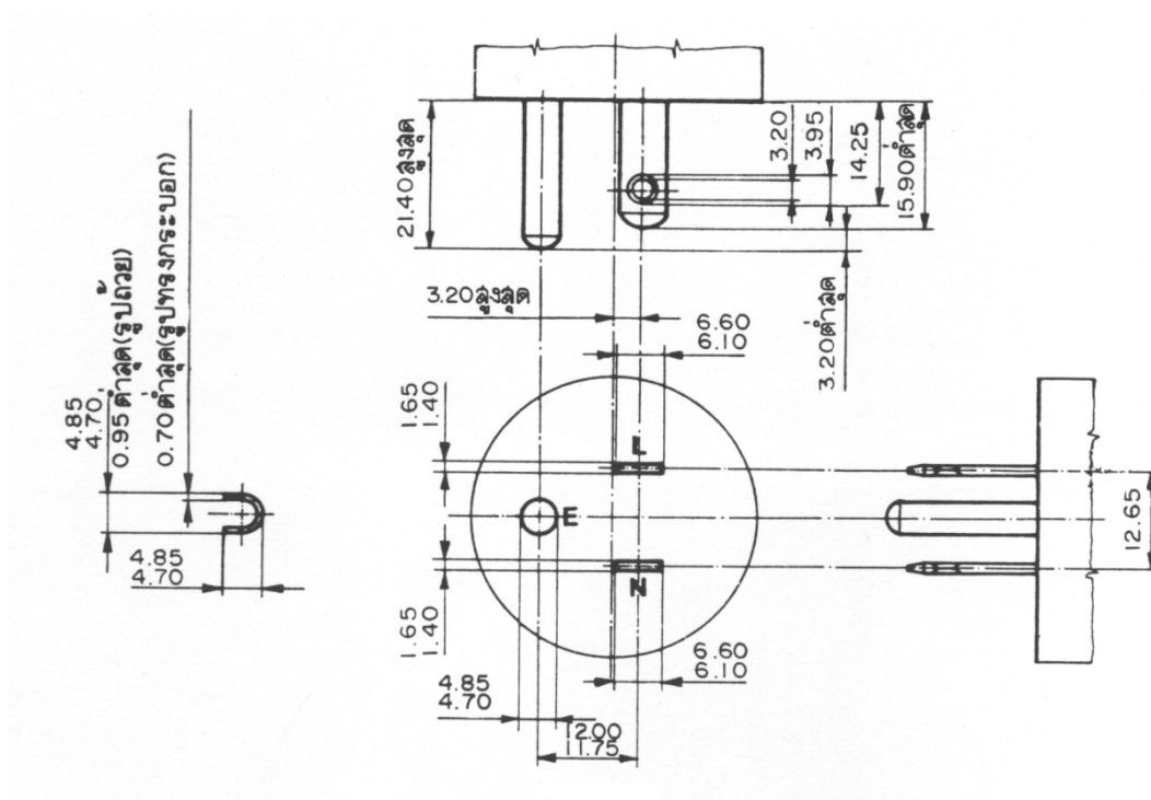
รูปที่ 101 ส่วนเด้าเสียบสองขั้วพร้อมขั้วสายดิน (แบบขาแบน)
