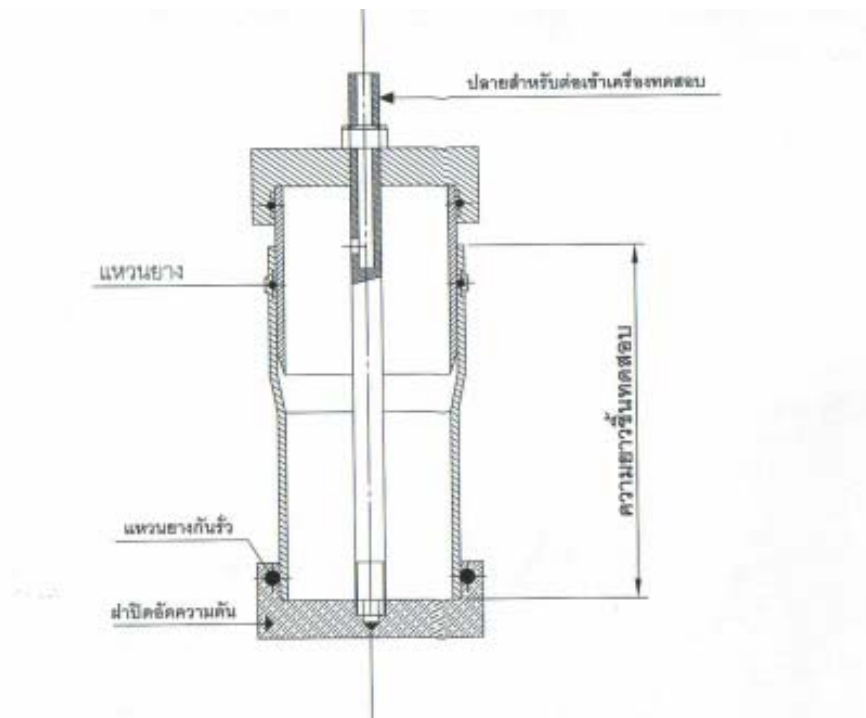
รูปที่ 3 การเตรียมชิ้นทดสอบสำหรับท่อปลายบานชนิดต่อด้วยแหวนยาง (ข้อ 11.8.2.2)
