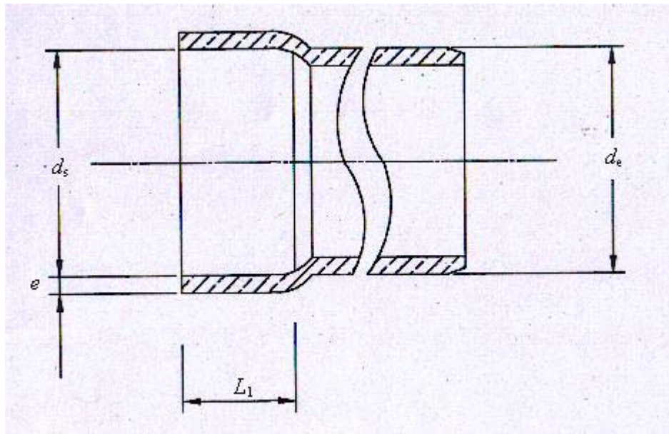
รูปที่ 1 มิติของท่อปลายบานชนิดต่อด้วยน้ำยา (ข้อ 6.2)
